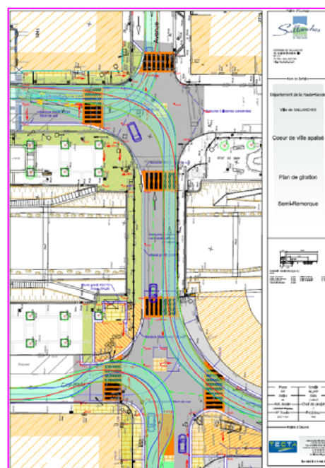
Plan de giration semi-remorque
